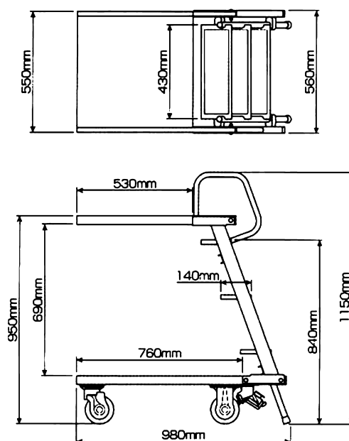
●寸法図
