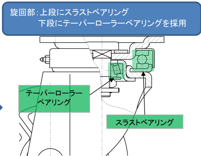
重荷重用キャスター RRJH-150
